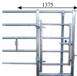
Handel med justerbar kalvpassage med port. Art nr. LV4 - 124256 Art nr. LV5 - 125295
