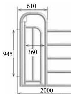
Handel med personpassage.
