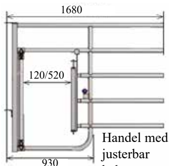
Handel med justerbar kalvpassage. Art nr. LV4 - 124255 Art nr. LV5 - 125290
