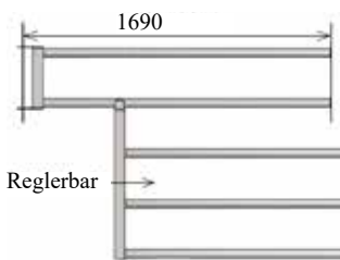
Handel med uttag för vattenho. Art nr. LV4 - 124240 Art nr. LV5 - 125300
